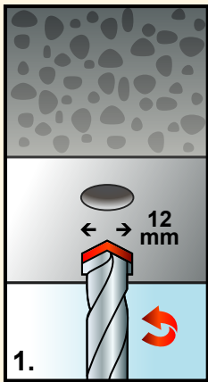
1. Percez 2 trous d'une profondeur de 7 cm. Foret diamant, diamètre 12mm.
