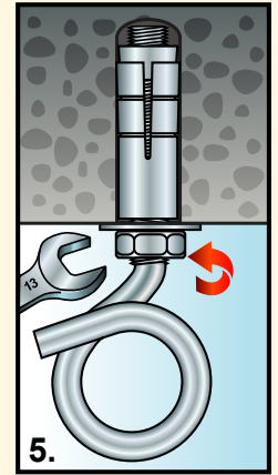
5. Serrer l'écrou avec un clé plate de 13 mm.
