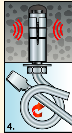
4. Visser le crochet jusqu'à la rondelle. Serrez fermement avec un tournevis.
